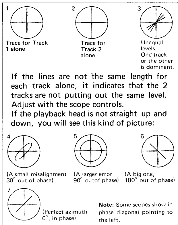
Fig. 2-23 Phase Shift
